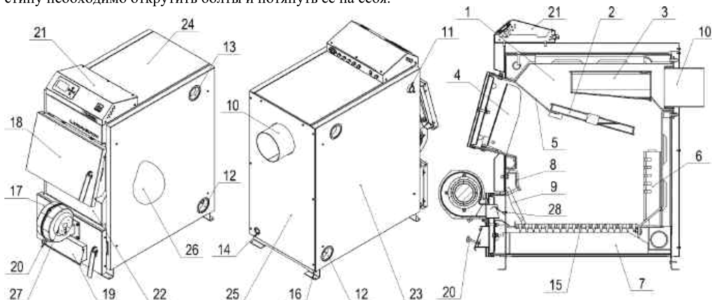
Рис. 2 Устройство котла
